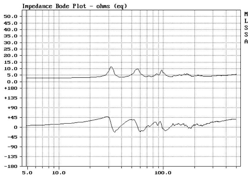
GAE EtaMax: Impedanzverlauf / Impedance plot @ 2 systems
