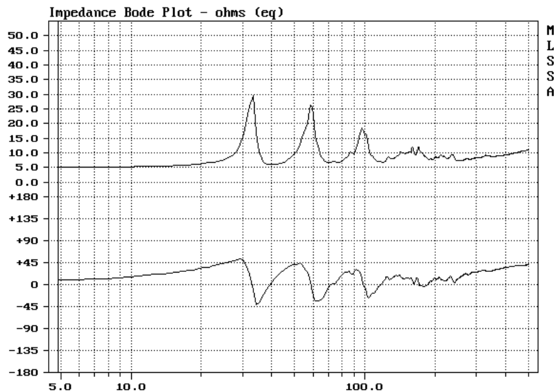
GAE EtaMax: Impedanzverlauf / Impedance plot @ 1 system
